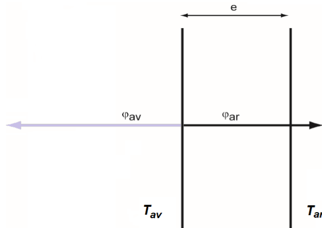
figure 6 – Flux thermiques au niveau du bouclier thermique
