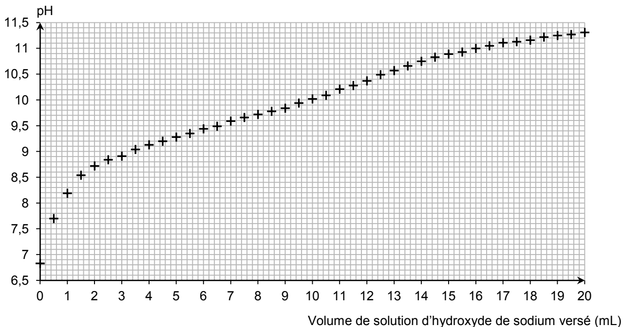
Figure 1. Titration de la solution suivi par pH-métrie.
