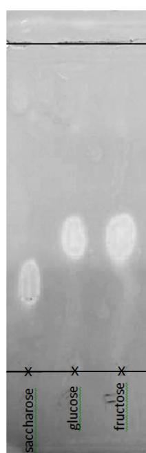
Photographie du chromatogramme
