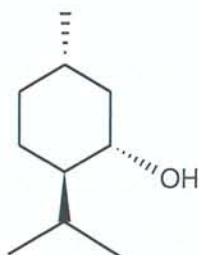
stéréoisomère 1
