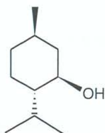
(-)-menthol
