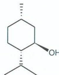
stéréoisomère 2
