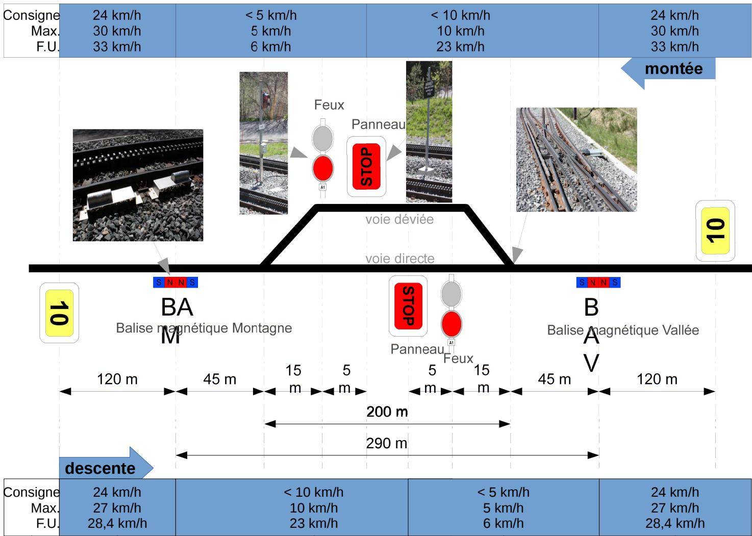
Figure 10 : schéma de conduite au croisement des Muletiers
