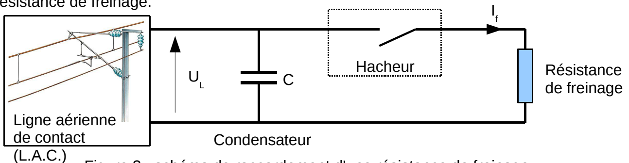
Figure 2 : schéma de raccordement d'une résistance de freinage
