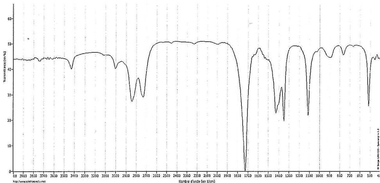
Document 2a : Spectroscopie Infrarouge en phase liquide. Spectre IR1
