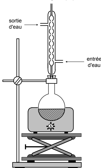
Figure 7. Schéma du montage expérimental
